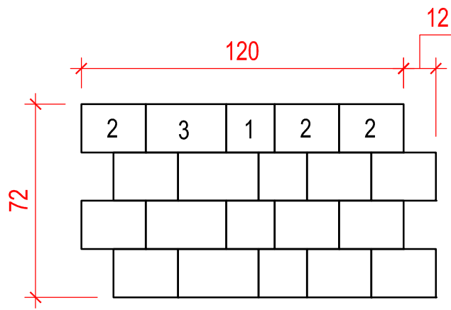
Form A mögliche Palettierung für Maschinenverlegung
