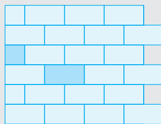
Läuferverband 60 x 30 cm, Anfänger 30 x 30 cm
