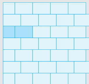
Läuferverband 60 x 40 cm, Anfänger 40 x 40 cm
