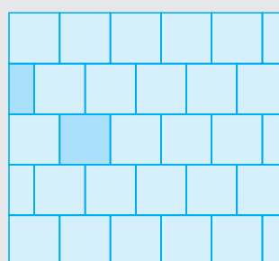
Läuferverband 60 x 60, Anfänger 60 x 30 cm
