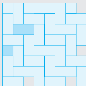
Fischgrätverband 60 x 30, Anfänger 60 x 30 cm bauseits halbiert
