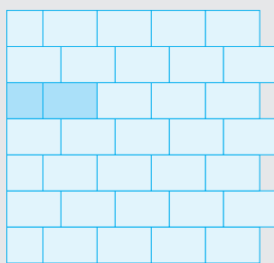
Läuferverband 60 x 40 cm, Anfänger 40 x 40 cm
