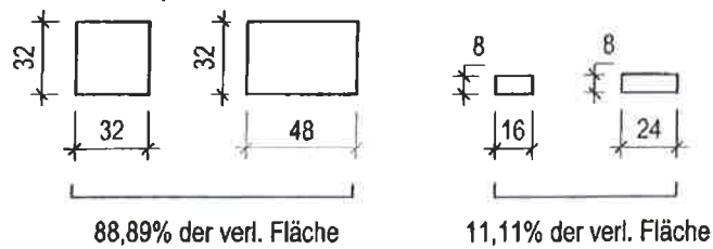
Bild: Tetrakron, Verlegebild Reihenverband V3
