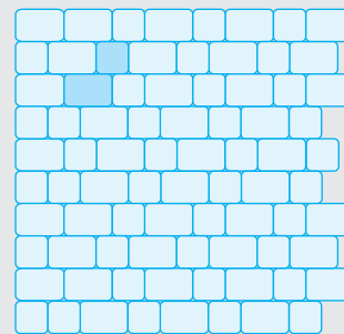
Systemverband gemischte Form 13,4 x 13,4; 20,1 x 13,4 cm
