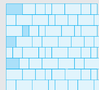
Gemischter Reihenverband mit 4 Formaten 26,25 x 17,5; 17,5 x 15,75; 21 x 17,5 und 17,5 x 10,5 cm
