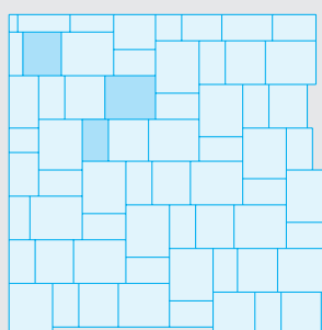
Wilder Verband "Muster 8" 17,5 x 10,5; 17,5 x 15,75 und 21 x 15,75 cm
