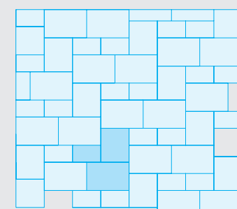
Verband Allgäu I 26,25 x 17,5; 17,5 x 10,5 und 21 x 17,5 cm
