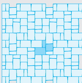
Wilder Verband mit 3 Formaten 12,6 x 6,3; 12,6 x 12,6; 18,9 x 12,6 cm
