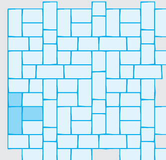
Wilder Verband mit 3 Formaten 12,6 x 12,6; 18,9 x 12,6; 25,2 x 12,6 cm
