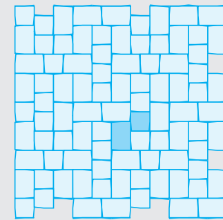
Wilder Verband mit 2 Formaten 12,6 x 12,6; 18,9 x 12,6 cm
