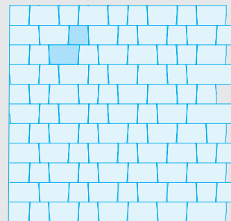
Gemischter Reihenverband mit 2 Formaten 12,6 x 12,6; 18,9 x 12,6 cm
