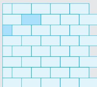
Läuferverband 31 x 17,5 cm
