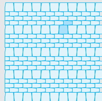
Streifenmuster mit 2 Formaten 12,6 x 6,3; 12,6 x 12,6 cm
