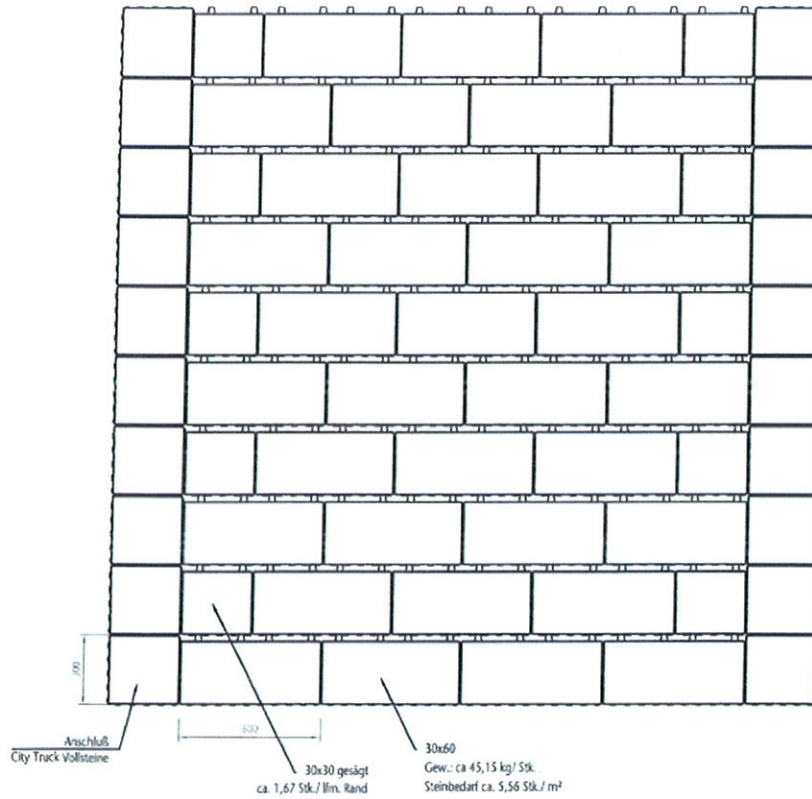
Bild: CityTruck Öko-Stein 60/30/12 mit 3 cm Längsfuge, Verlegebild
