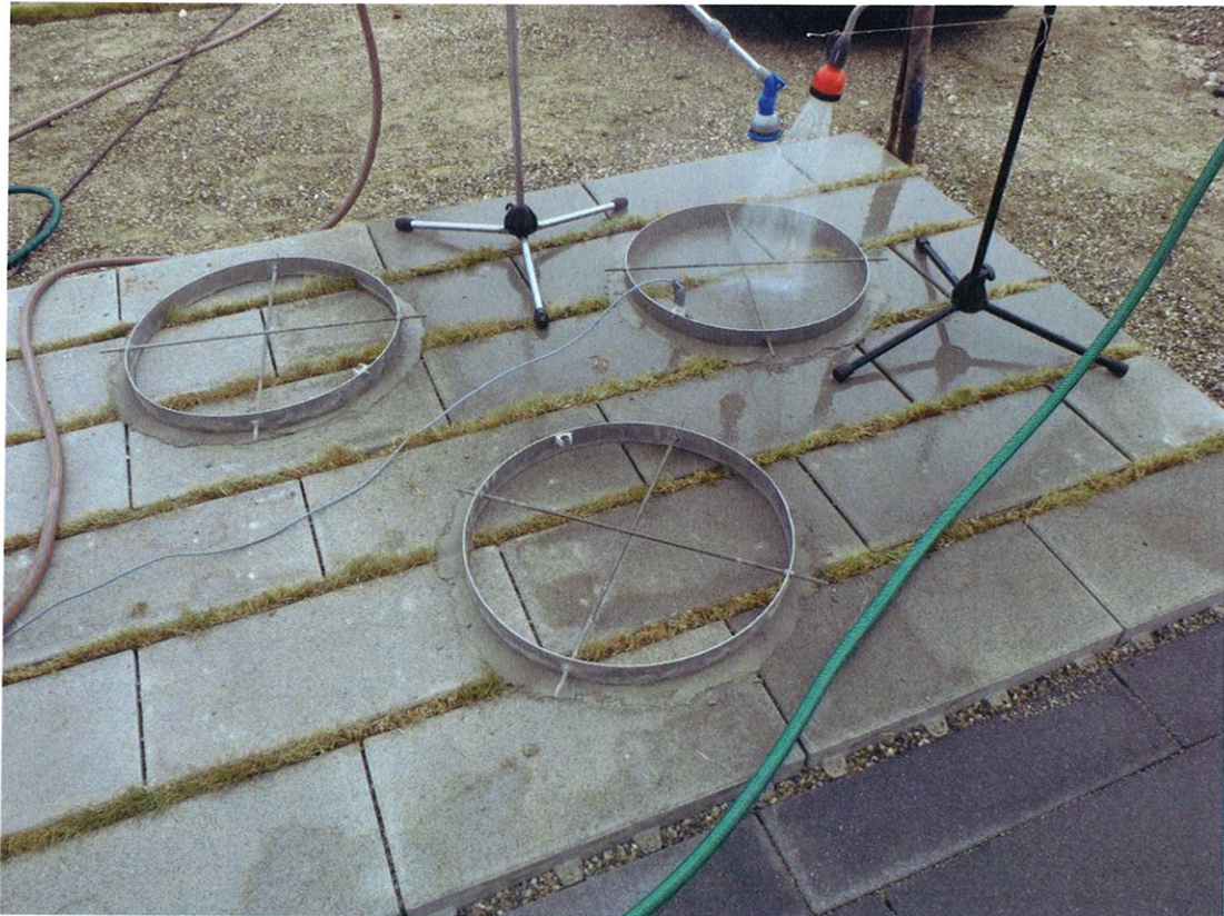
Bild: CityTruck Öko-Stein 60/30/12 mit 3 cm Längsfuge
